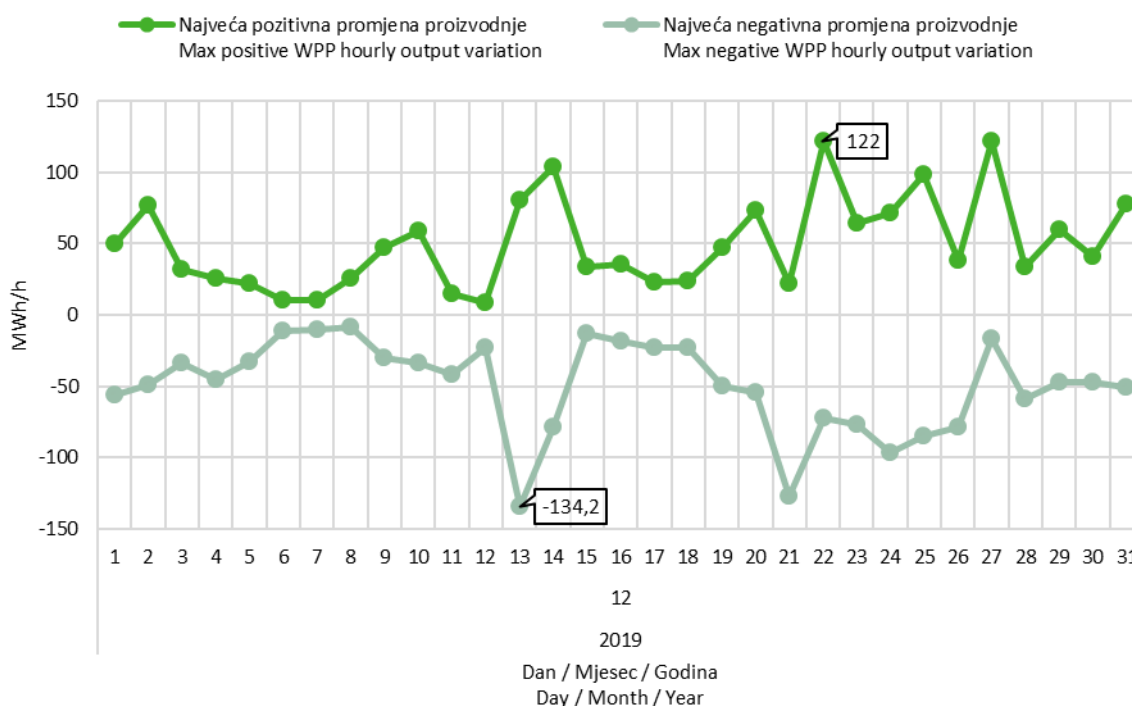
Slika 9 Maksimalna pozitivna i maksimalna negativna promjena satne proizvodnje VE u prosincu 2019. godine
