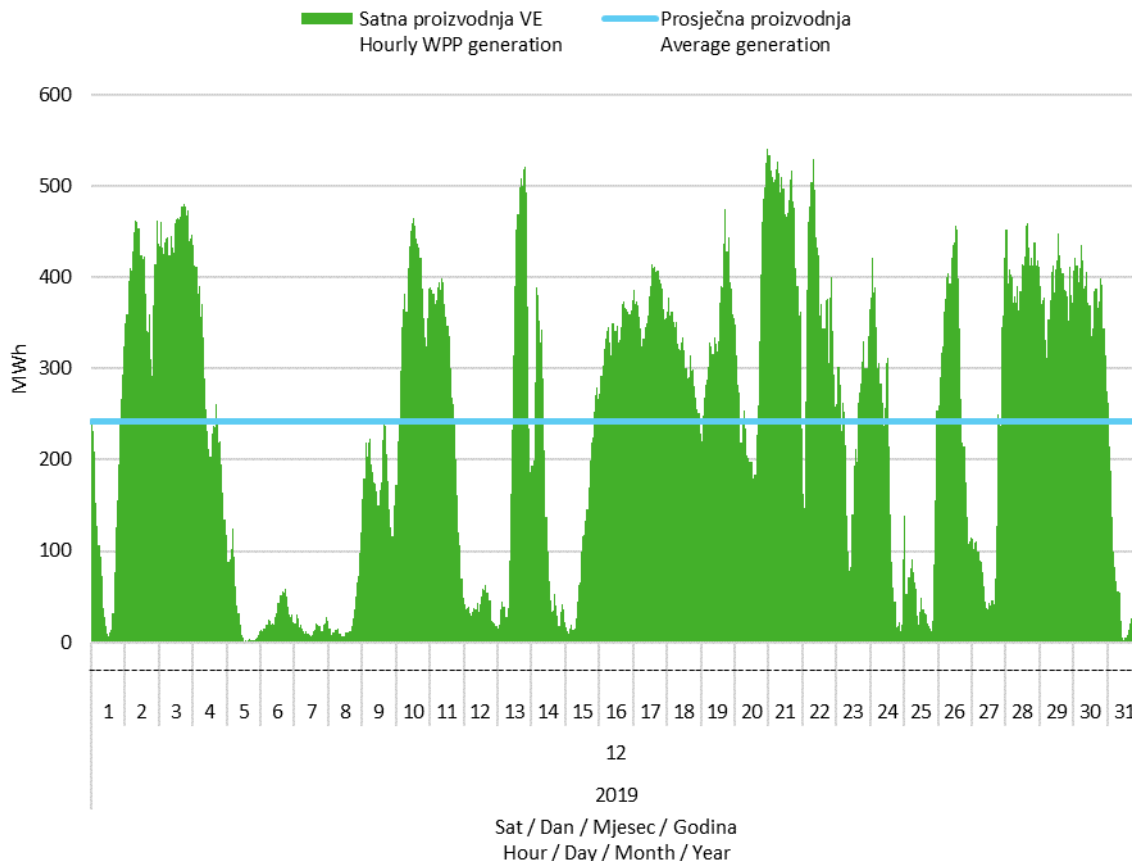
Slika 2 Satna proizvodnja svih vjetroelektrana u prosincu 2019. godine
