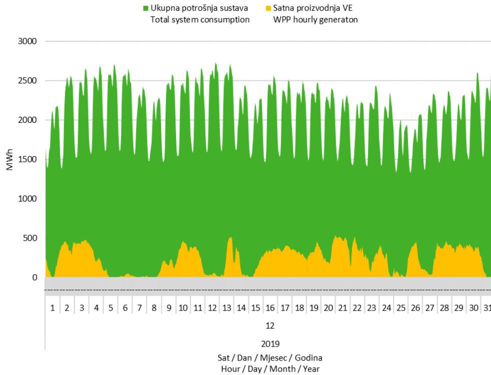
Slika 7 Usporedba satnog dijagrama opterećenja sustava i proizvodnje vjetroelektrana u prosincu 2019. godine
