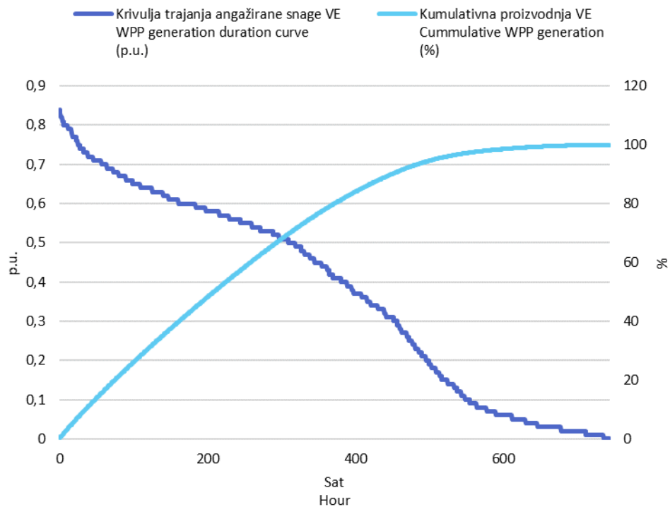
Slika 3 Krivulja trajanja angažirane snage svih VE i kumulativna proizvodnja VE u prosincu 2019. godine u jediničnim vrijednostima
