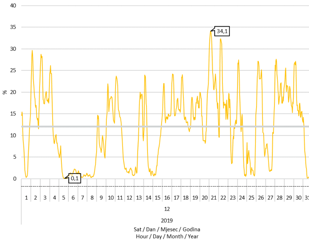
Slika 8 Udio proizvodnje vjetroelektrana u pokrivanju satnog opterećenja elektroenergetskog sustava u prosincu 2019. godine
