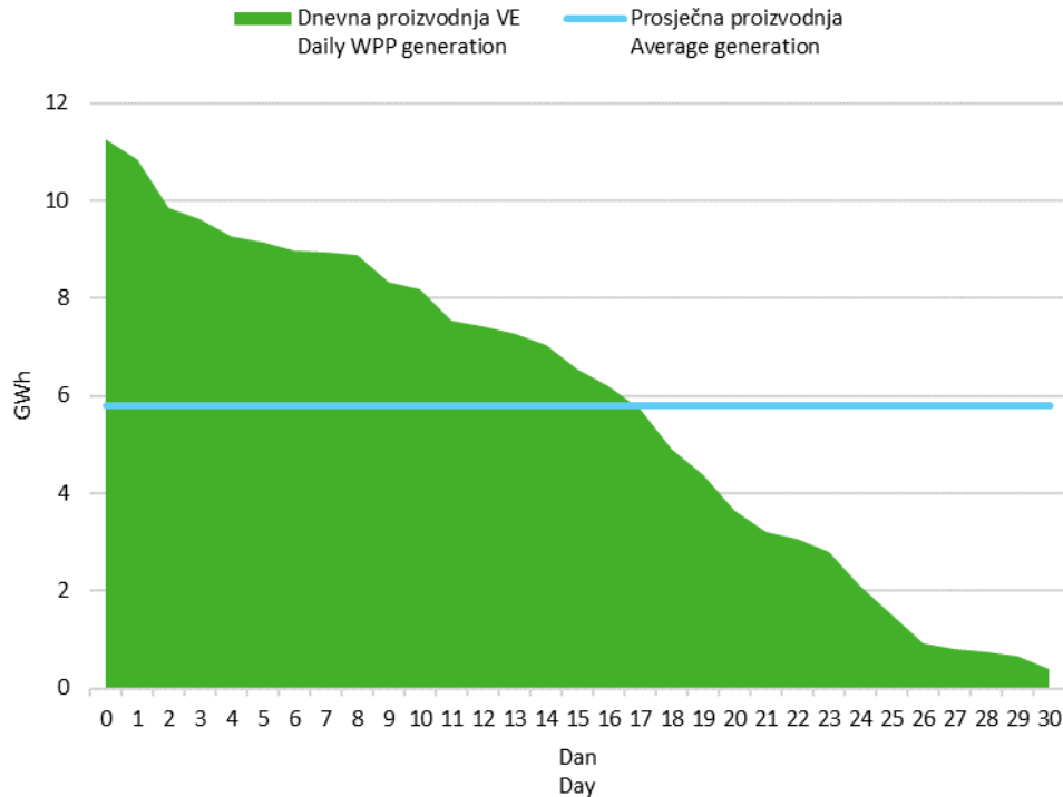
Slika 6 Krivulja trajanja dnevne proizvodnje vjetroelektrana u prosincu 2019. godine
