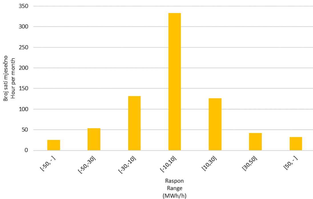
Slika 10 Statistička raspodjela satnih promjena proizvodnje VE u prosincu 2019. godine
