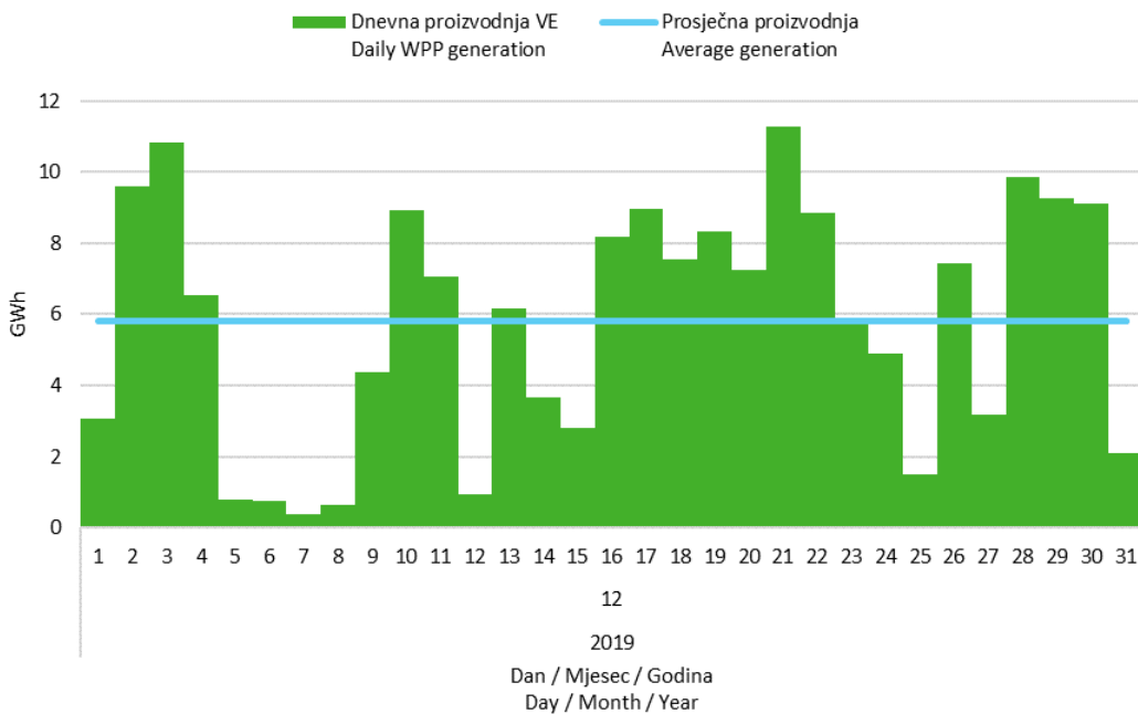
Slika 5 Dnevna proizvodnja svih vjetroelektrana u prosincu 2019. godine Figure 5 Daily generation of all wind power plants in December 2019
